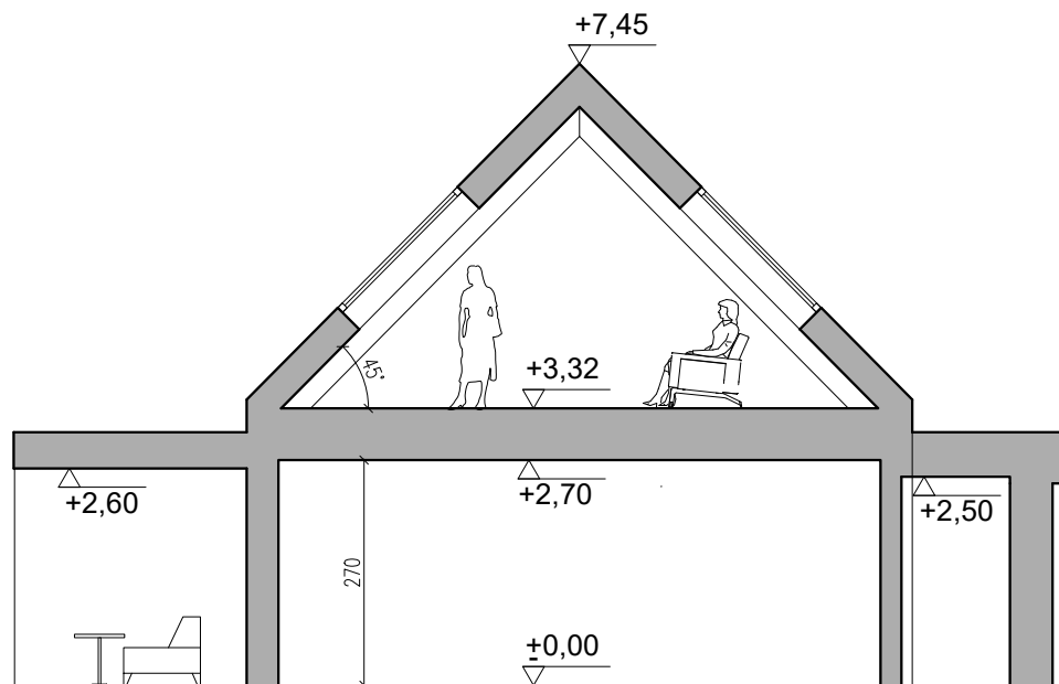
Przekrój
